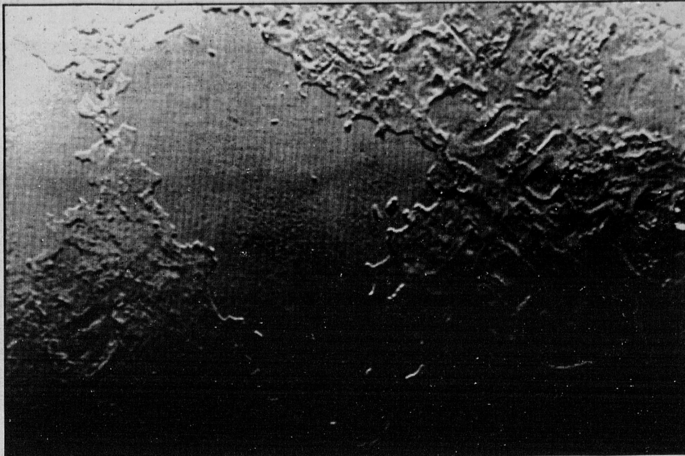
Yksityiskohta Tritonin pinnalta osoittaa, kuinka erinomaista kuvamateriaalia Voyager 2 pystyi Maahan välittämään. Kuvaa hallitseva allas on noin 200 kilometriä leveä ja 400 km pitkä. Altaan alareunassa erottuvat heikosti kahden muinaisen tulivuoren kraatterit, joiden reunat ovat sortuneet altaan aikanaan täyttäneeseen nesteeseen. Tämäkin kuva todistaa tritonin pinnan nuoruutta: toisten kappalaiden törmäyksessä syntyviä kraattereita ei ole.
