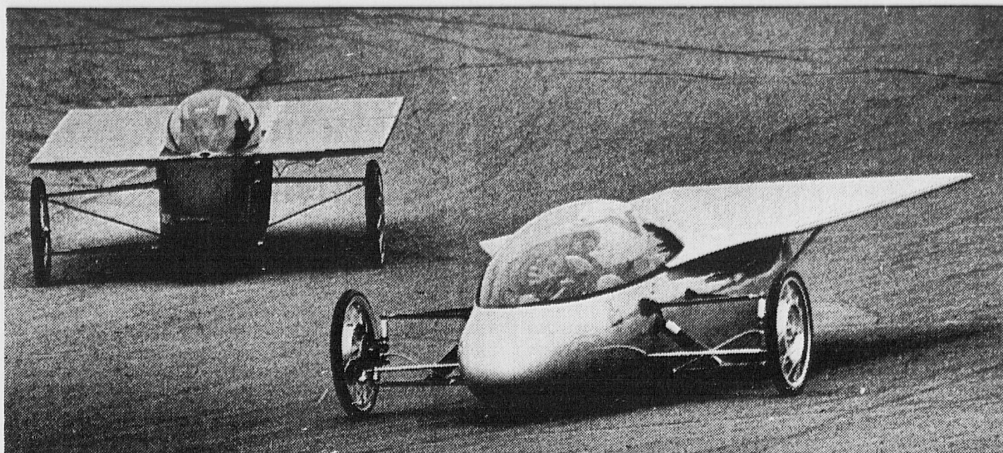
Aurinkoenergialla toimivat kilpa-autot testauskierroksellaan. Autot syntyivät MIT:n ja Dartmouth Collegen oppilaiden yhteistyön tuloksena.
