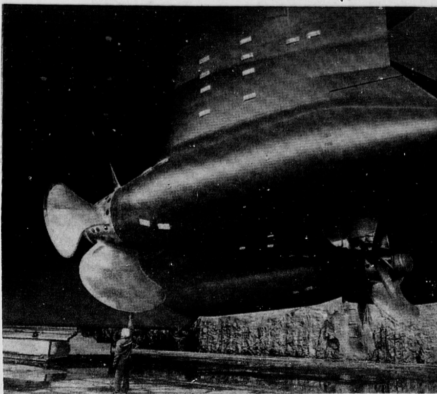
Tällaiset ruoripotkurit, jotta laivassa tulee olemaan kolme, vievät aluksen eteenpäin. Pituutta on 11 metriä, painoakin reilut 170 tonnia kappaleita. Kuvassa mies näyttämässä putteet.
